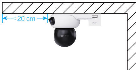
Fig. 2 Vägghermonterong
