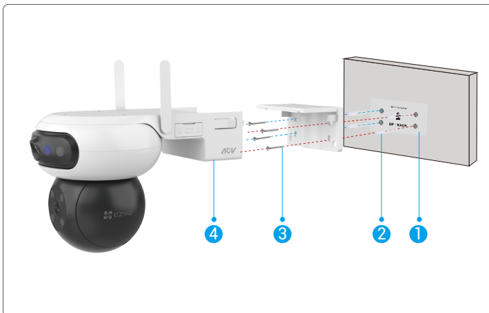
Fig. 2 Vägghermonterong
